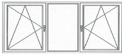
Kippi-kiinteä (MSEY2/MEK_VK)
